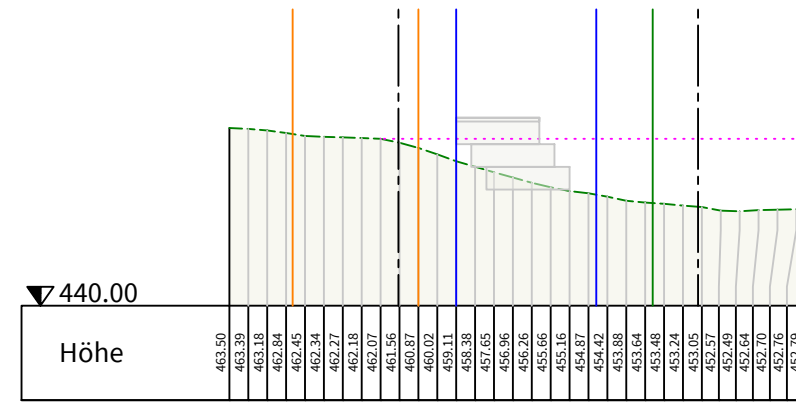
Geländeschnitt 5 - 5
