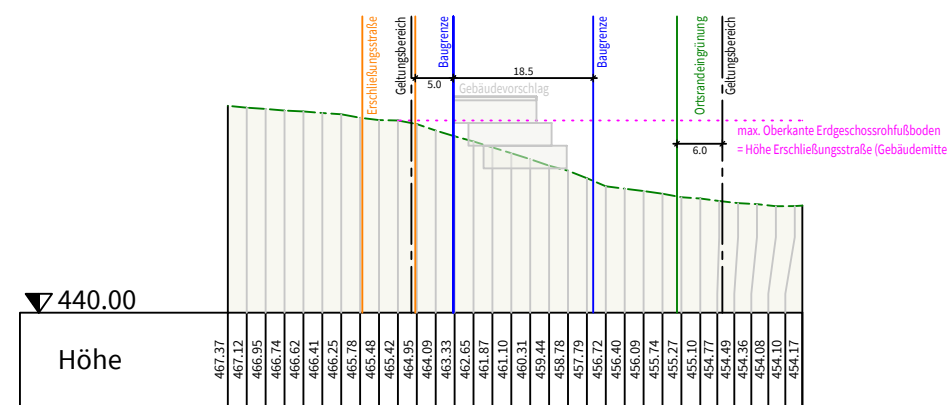
Geländeschnitt 1 - 1
