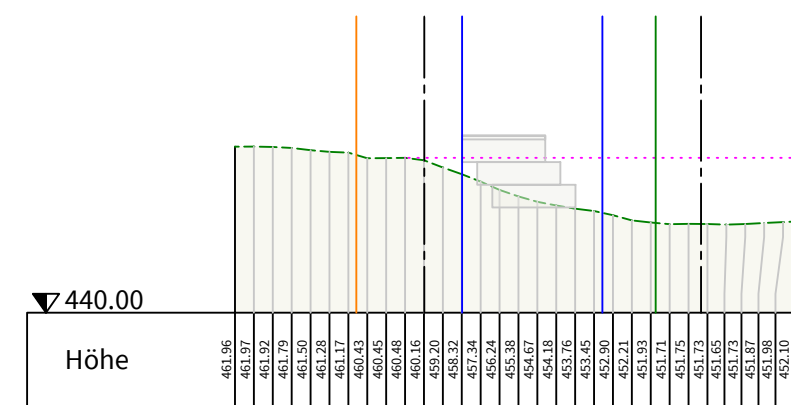
Geländeschnitt 7 - 7
