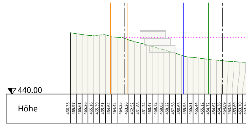
Geländeschnitt 2 - 2
