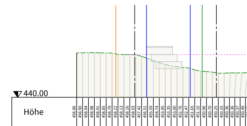
Geländeschnitt 10 - 10
