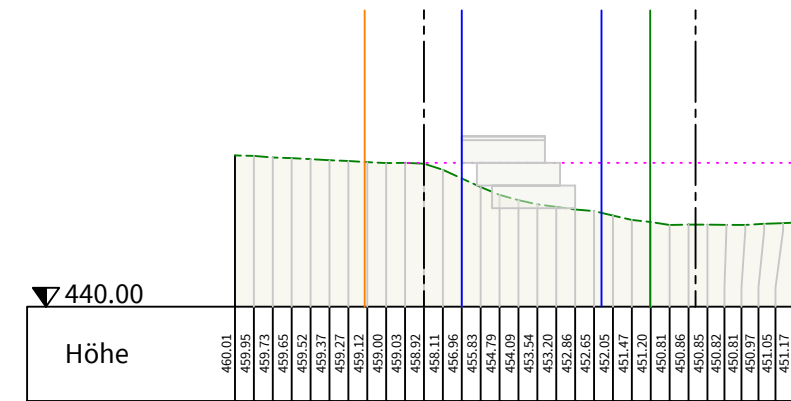
Geländeschnitt 9 - 9
