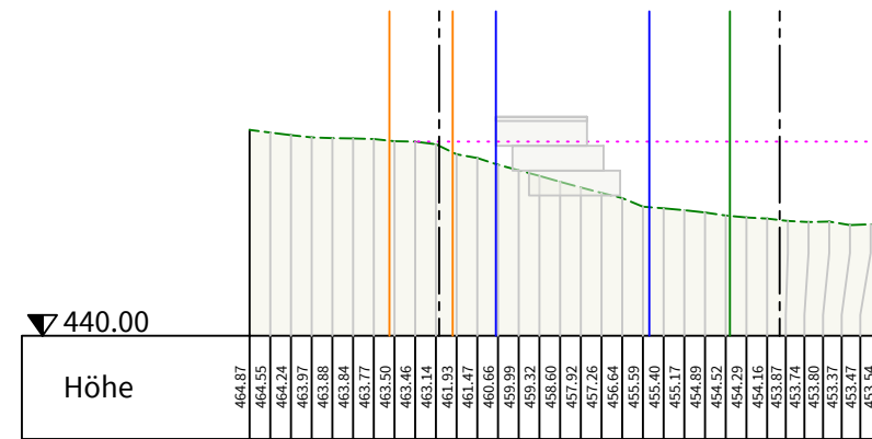
Geländeschnitt 3 - 3
