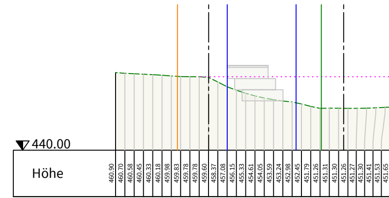
Geländeschnitt 8 - 8
