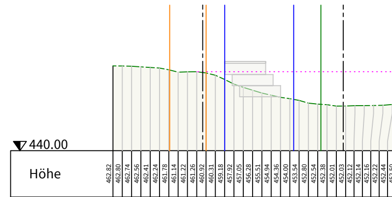
Geländeschnitt 6 - 6
