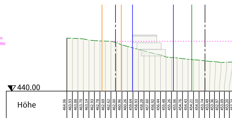
Geländeschnitt 4 - 4
