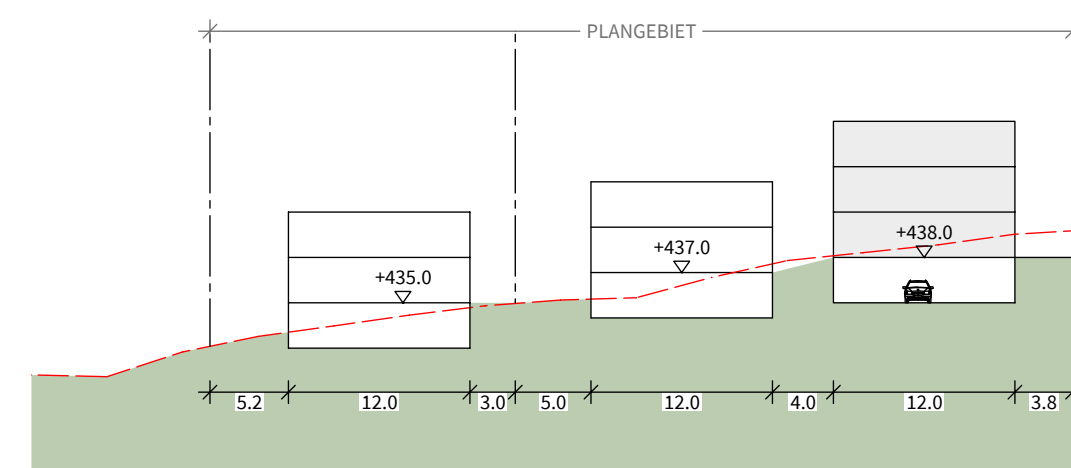
Schnitt 12-12
